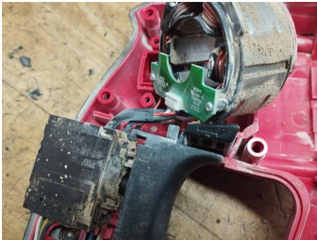
Obr.2 Zanesenie nečistôt na statore a spínači
