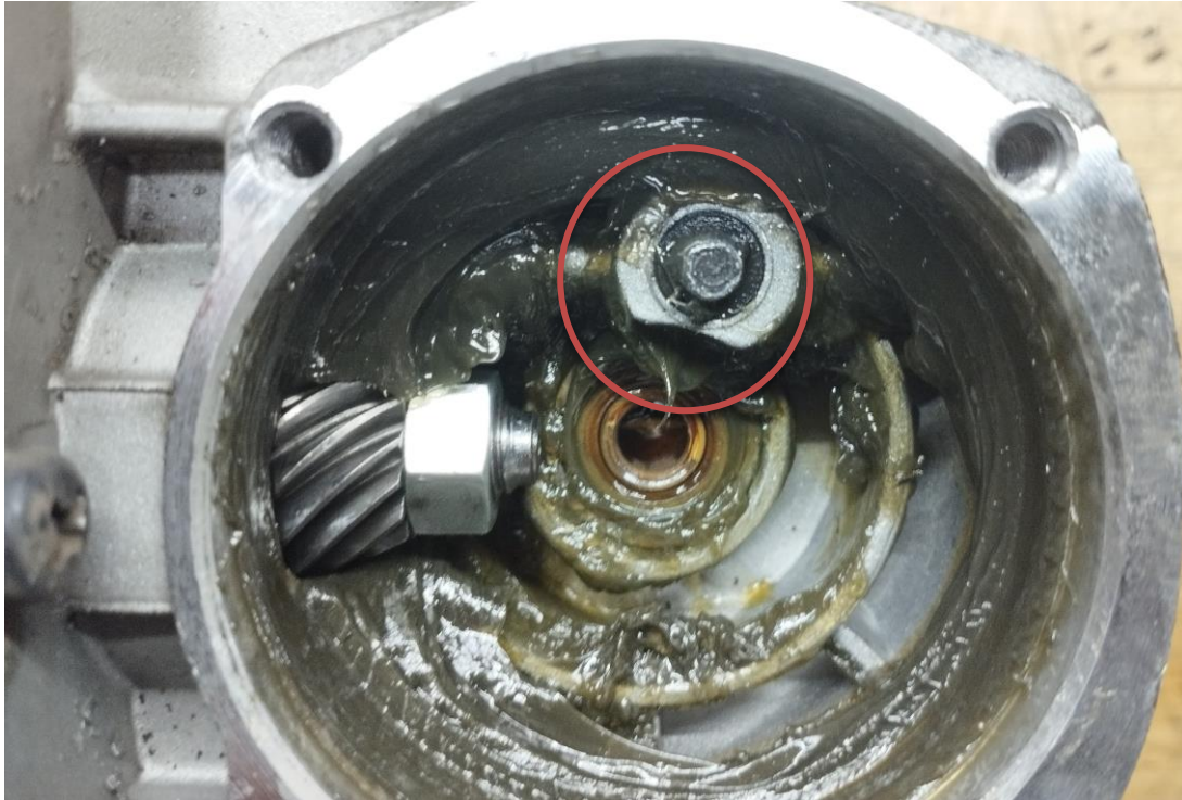
Obr.1 Poškodenie aretačného kolíka
