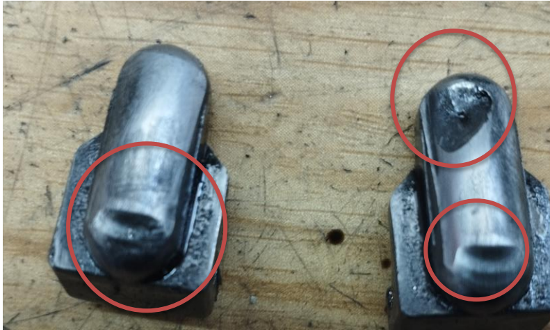
Obr.4 Poškodenie valčekov upínania
