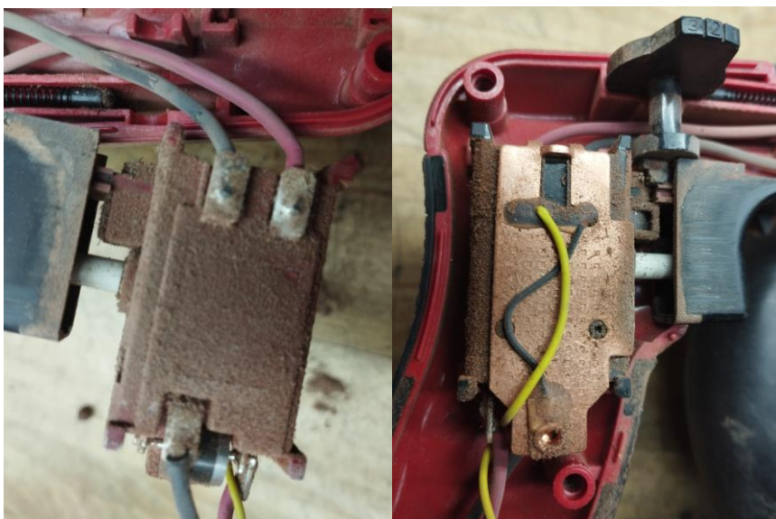
Obr.2 Znečistenie spínača
