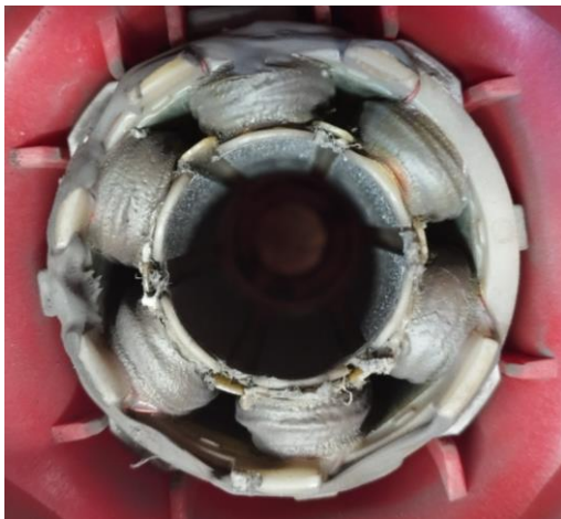
Obr.2 Poškodenie statora
