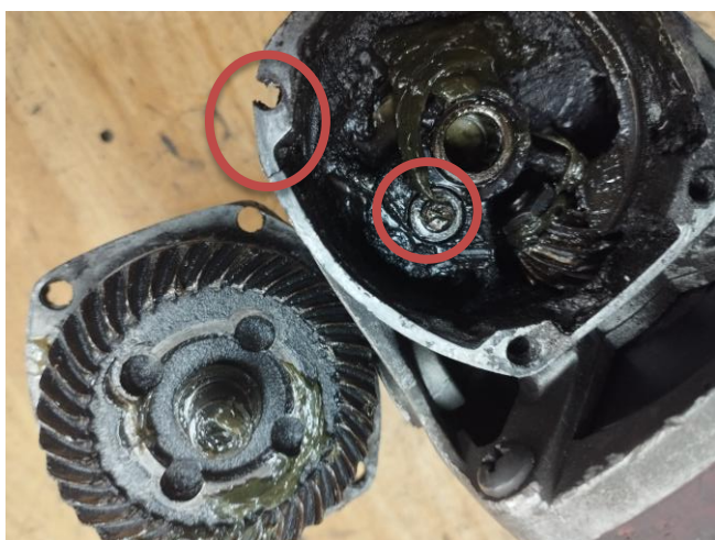
Obr.3 Poškodenie puzdra prevodovky, aretácie kotúča a opotrebovanie ozubených prevodov
