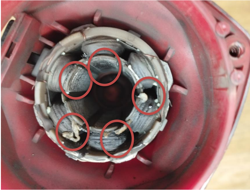
Obr.4 Poškodenie statora
